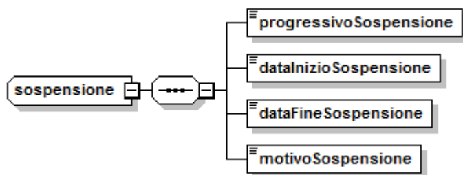
Figura 7 - FILE2 nodo Sospensione
