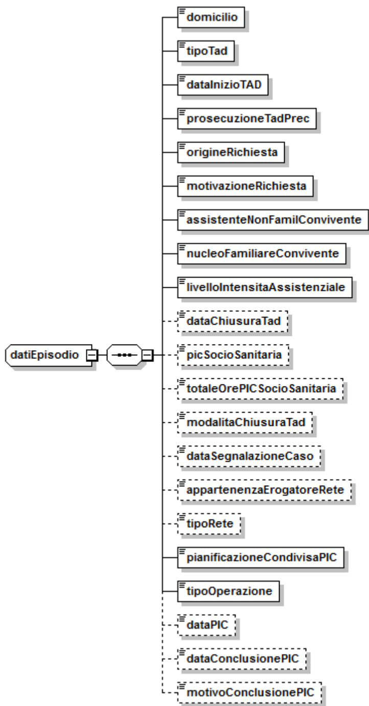
Figura 4 - FILE2 nodo Dati episodio di cura
