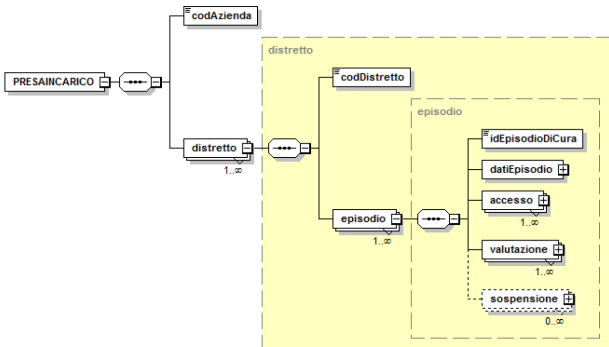
Figura 3 - FILE2 Presa in carico
