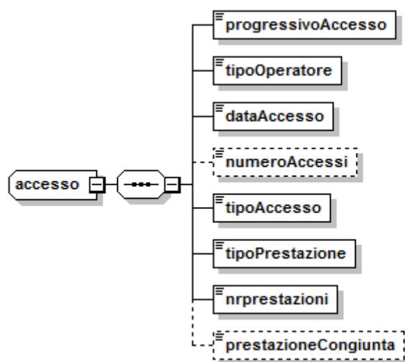
Figura 5 - FILE2 nodo Accesso
