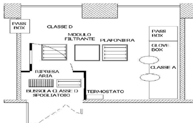
Figura 100S Piantina del locale classificato
